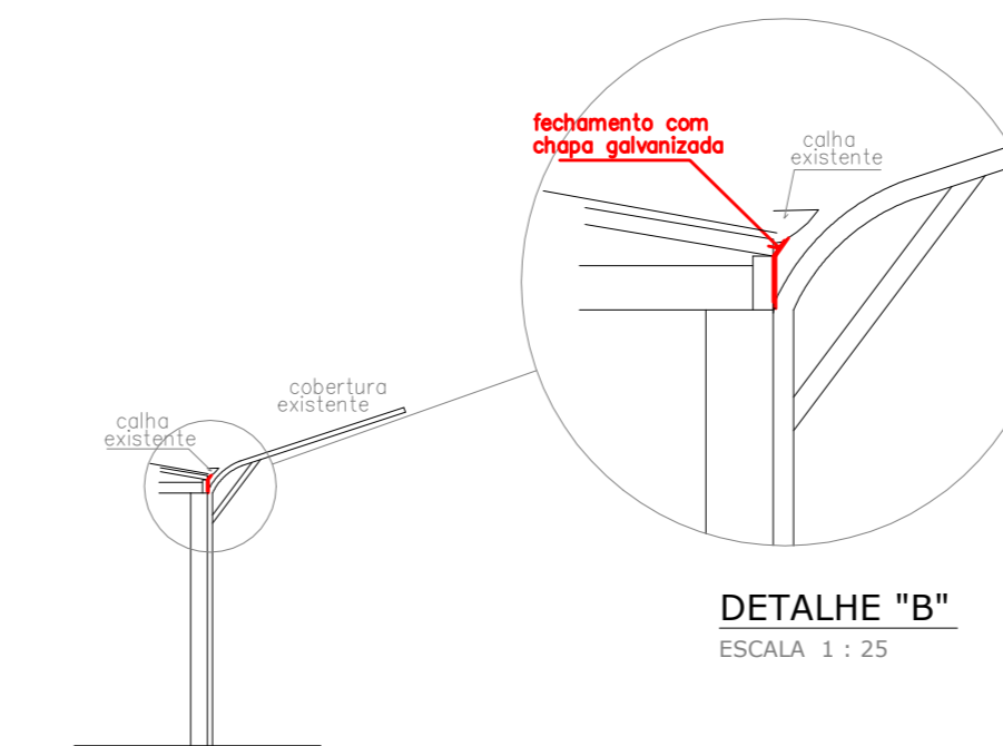
PERFIL ESCALA 1 : 100
