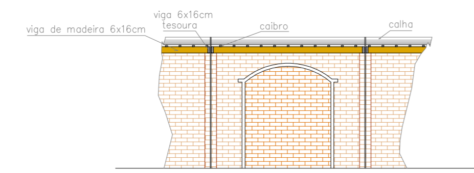
FACHADA EXISTENTE ESCALA 1 : 100
