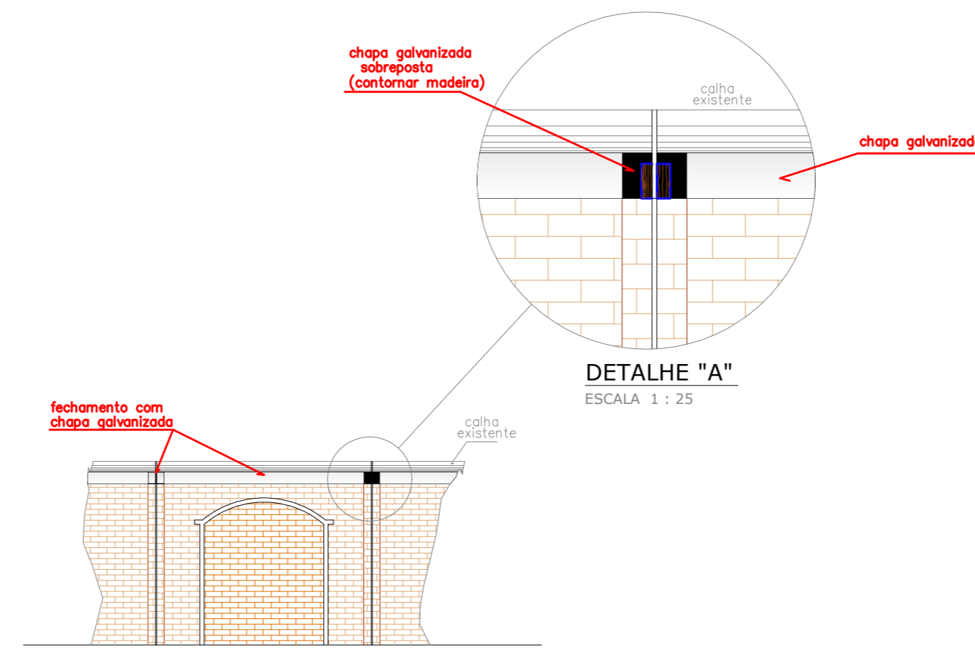
FACHADA PROPOSTA ESCALA 1 : 100
